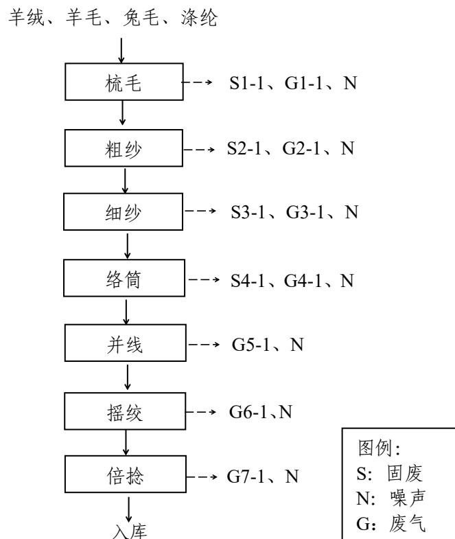
图 1-1 现有项目产品工艺流程图
