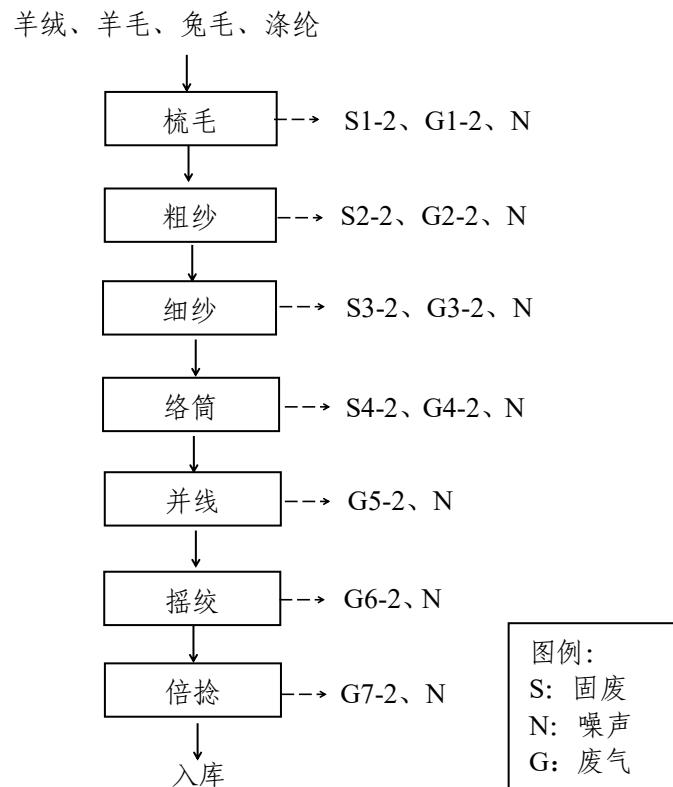
图 5-1 项目工艺流程图
